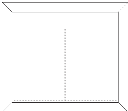
Art.nr: 105510445 alt. 106510445 Namnarksremsor 19stx13mm alt. 13stx19mm samt insticksficka med plats för 1st A4.
